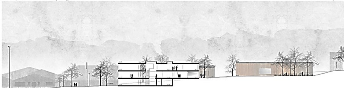
coupe transversale sur le bâtiment de l'enseignement
